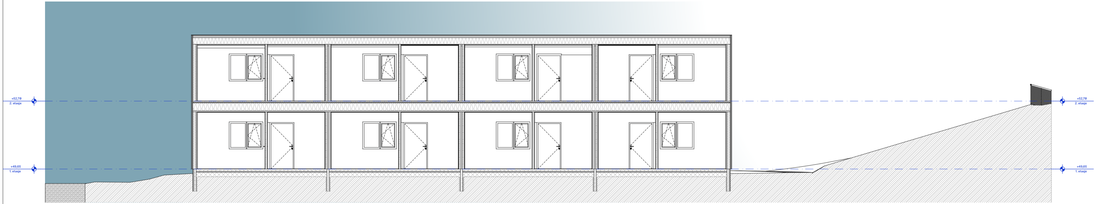
1:100 Snitt A
