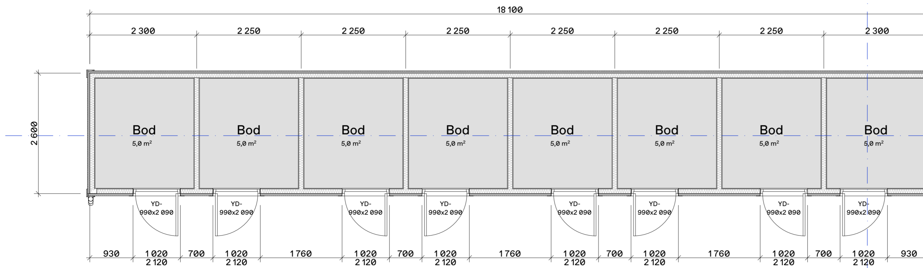
1. etasje
