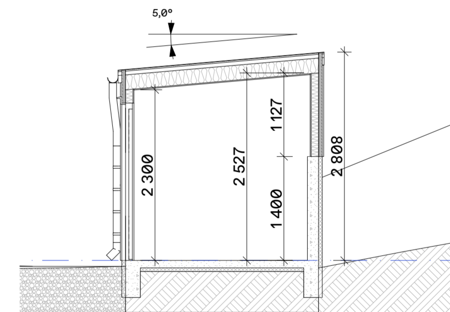
Snitt A
